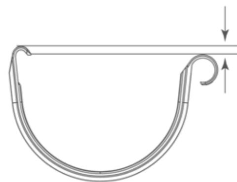
Рис. 1. Поперечное сечение желоба.
